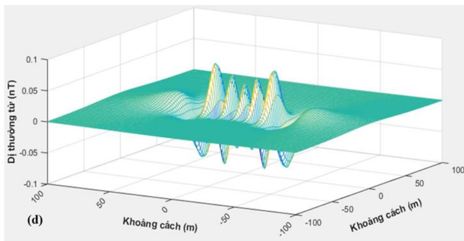
Phân bố bù dị thường từ của cửa vỏ tàu sau khi bù theo thuật toán Interior-Point.
