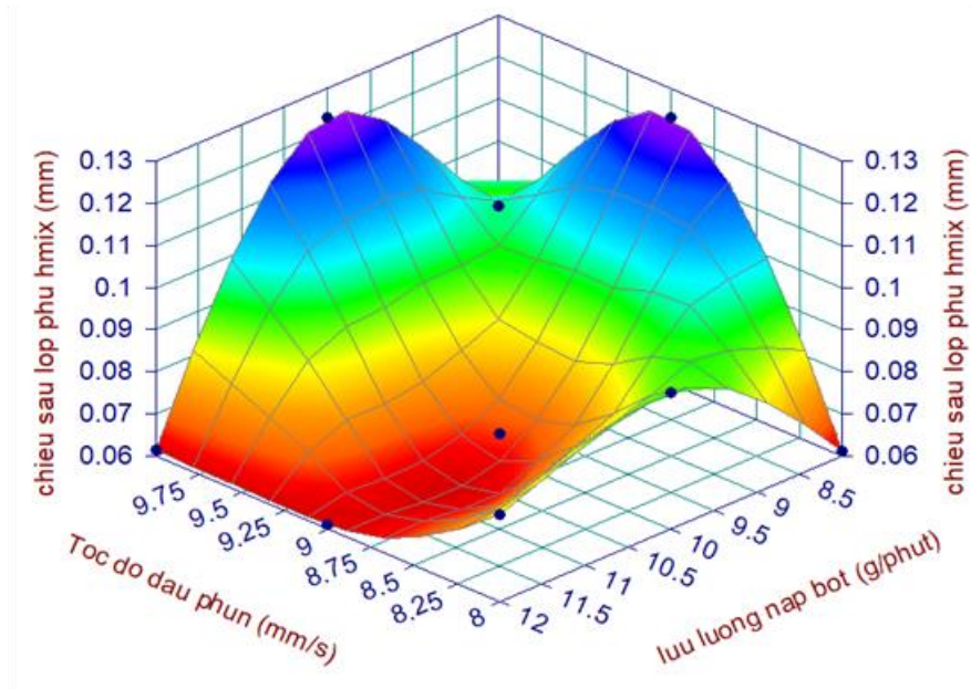
Mối quan hệ giữa các thông số công nghệ với chiều sâu lớp tạo hình.
